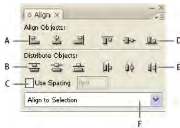
Align panel
