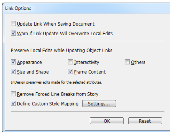
Link Options
